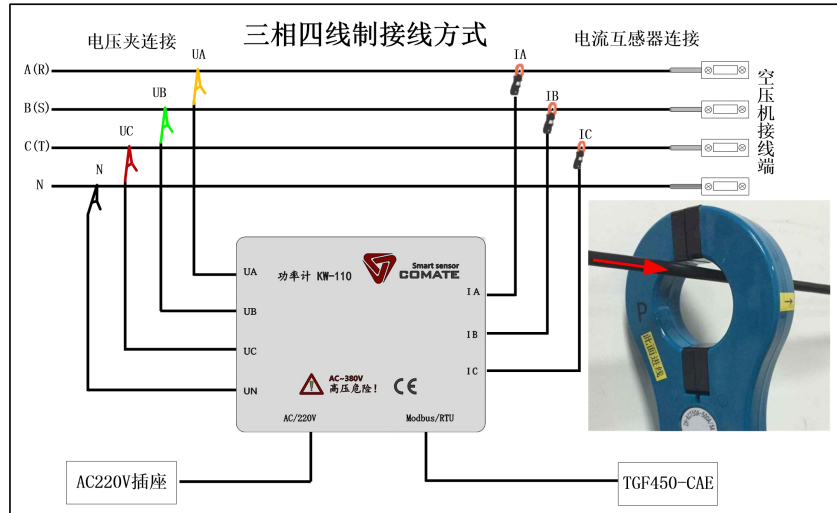
图 3.2.2 三相四线制接线图
