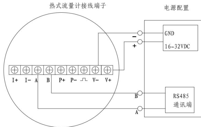
图 3.5 TGF450RS485 接线
