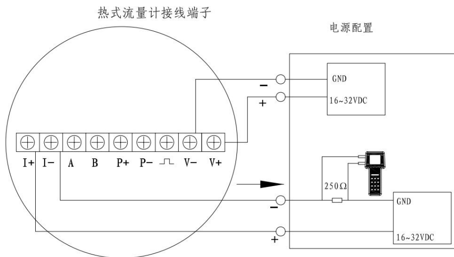
图 3.4 TGF450 四线制 Hart@4~20mA 输出
