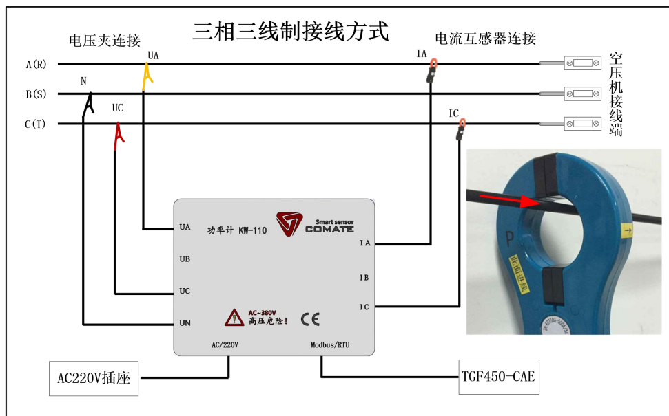
图 3.2.1 三相三线制接线图
