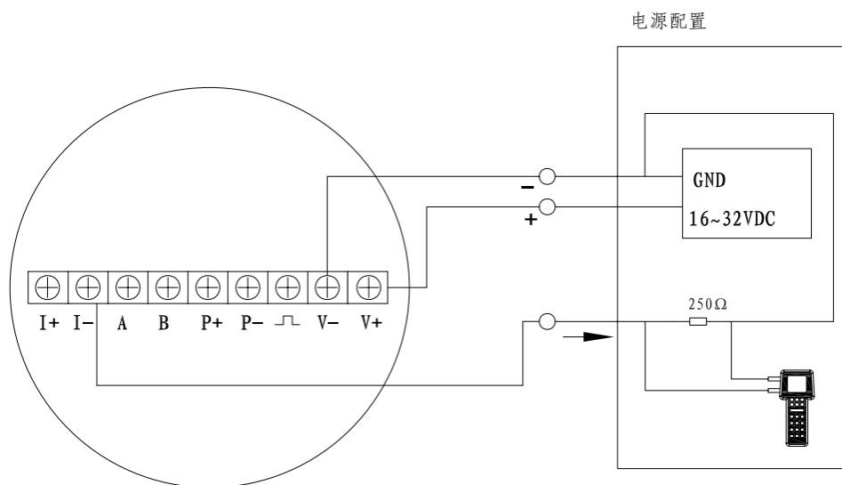
图 3.3 TGF450 三线制 Hart@4~20mA 输出
