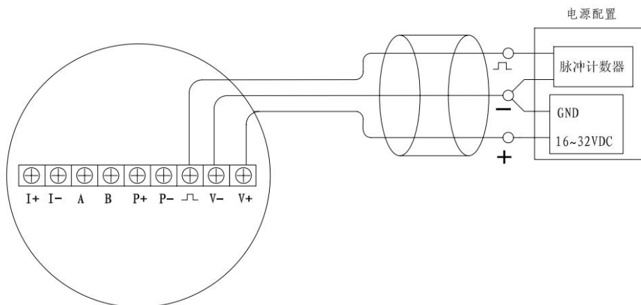
图 3.2 TGF450 三线制脉冲输出
