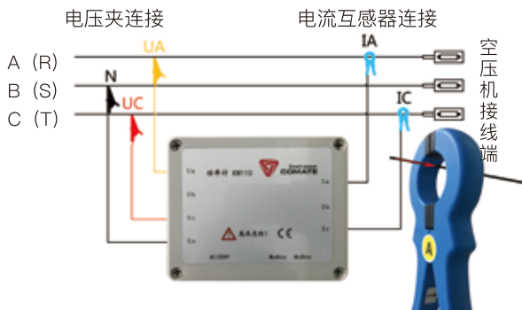
图3.7.1 三相三线制接线图
