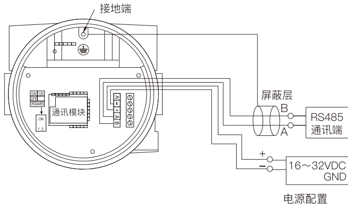
图3.5.2 RS485接线
