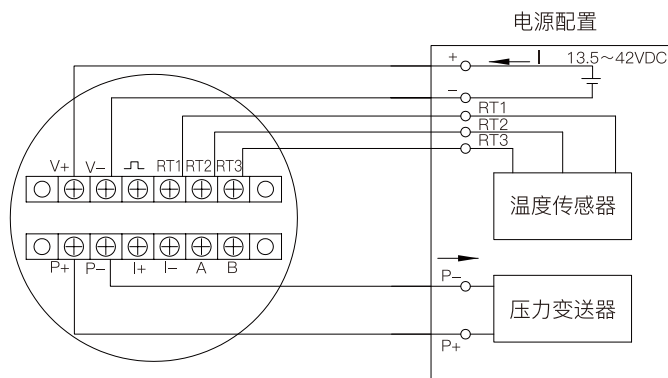
图3.4.5 外置式温度、压力接线示意图
