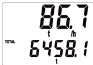
图4.3 蒸汽质量流量的瞬时量和累积量
