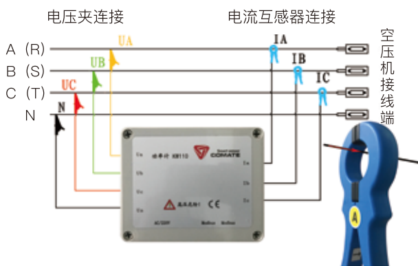
图3.7.2 三相四线制接线图
