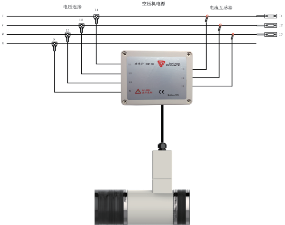
图 3.2.1 CAE350S接线图
