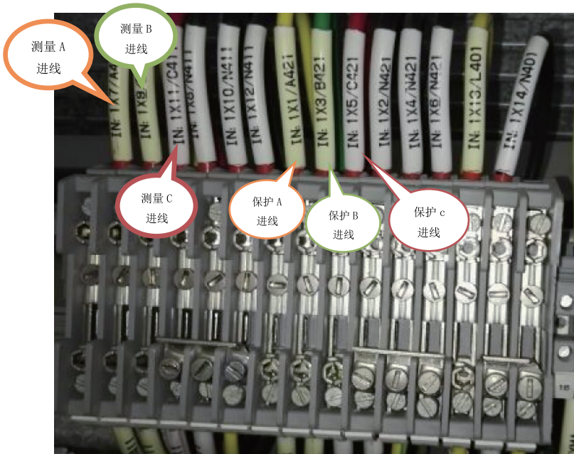
图6.2 三相电流
