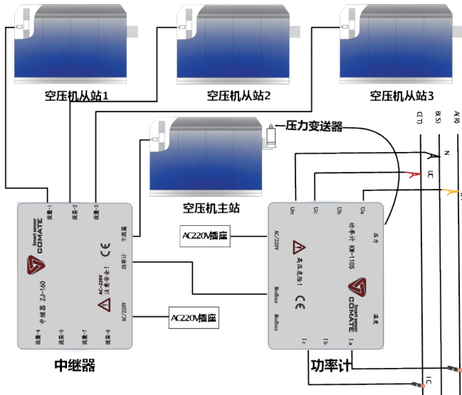
图5.1 空压站接线
