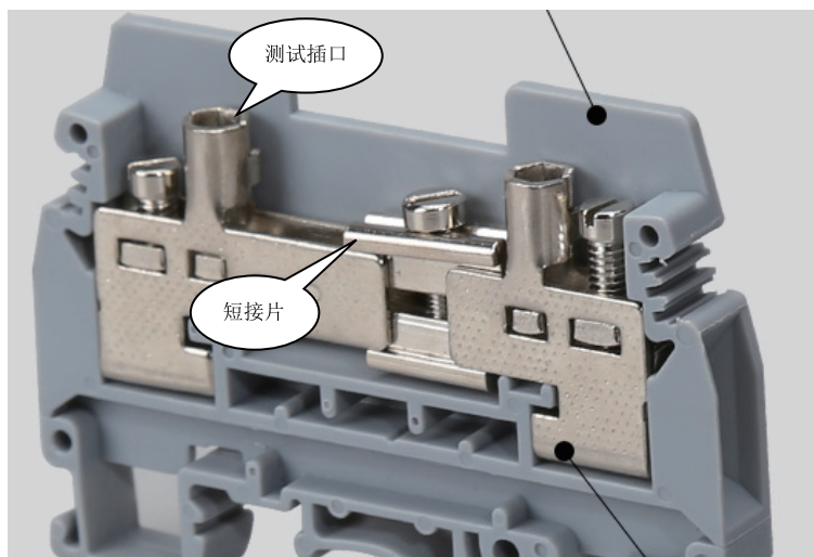
图6.4 电流端子侧视图
