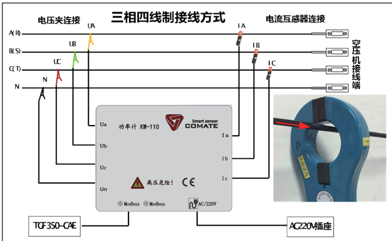
图 3.1.2 三相四线制接线图
