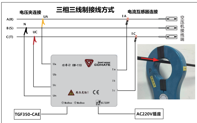
图 3.1.1 三相三线制接线图
