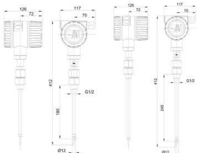
探杆长度为255mm尺寸图
