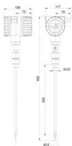
探杆长度为395mm尺寸图
