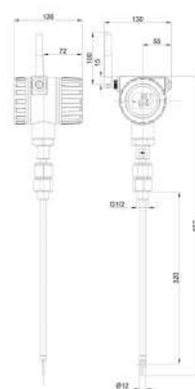
探杆长度为395mm尺寸图
