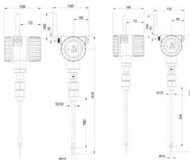
探杆长度为255mm尺寸图
